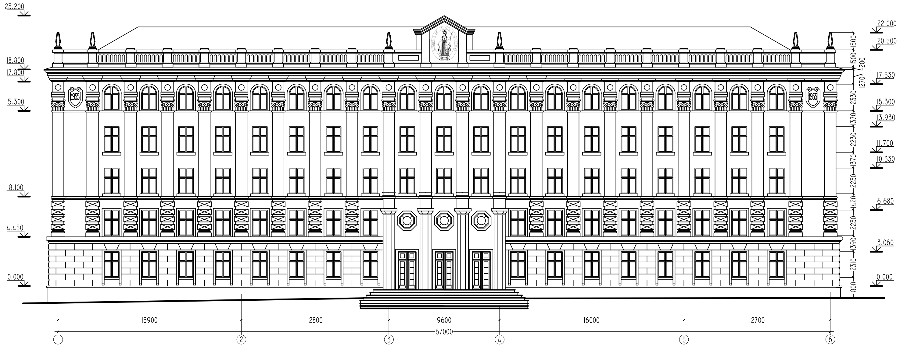
Façada în axe 1-6 Sc. 1: 200
